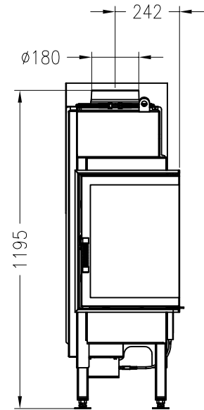
Seitenansicht M~1:20
