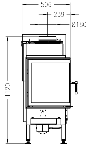
Seitenansicht M~1:20
