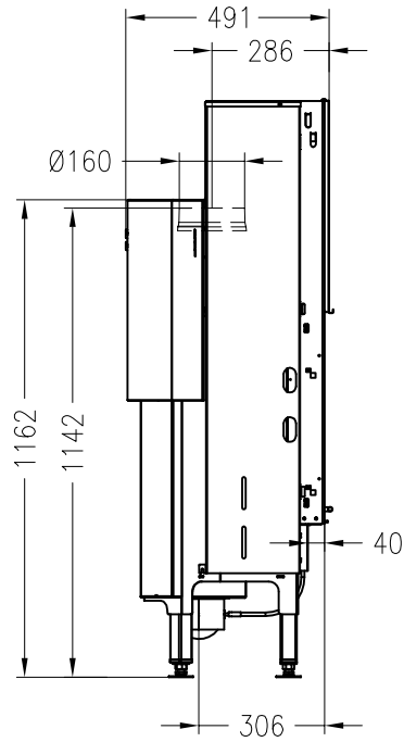
Seitenansicht M~1:20
