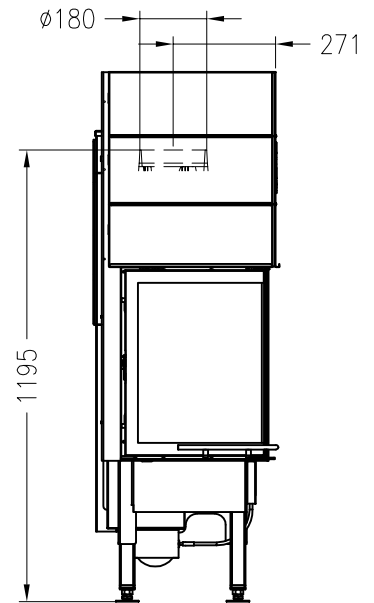
Seitenansicht M~1:20
